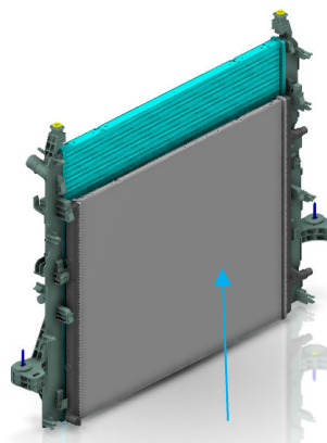
Refrigeração de sobrealimentação
